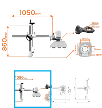
Specjalne podpory
