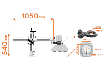
Specjalne podpory
