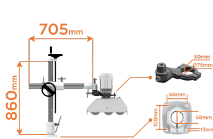
Specjalne podpory
